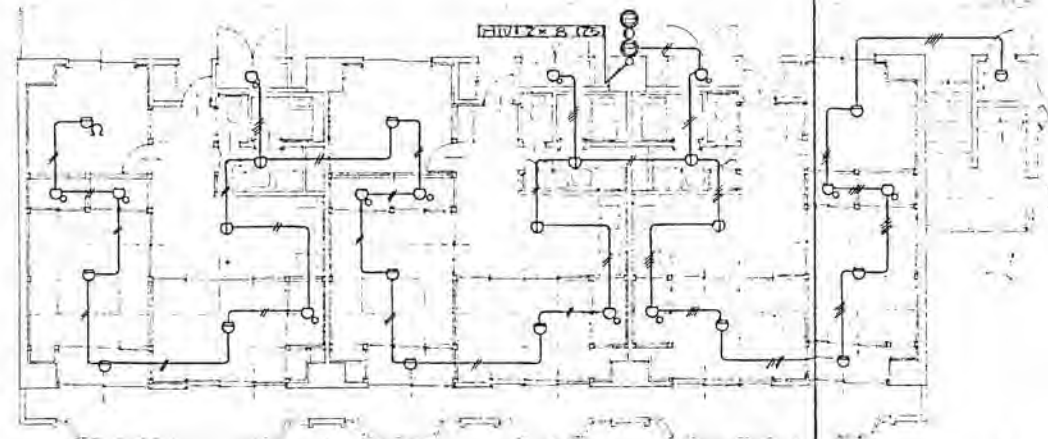
5階平面図
