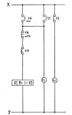
ポンプ制御回路
