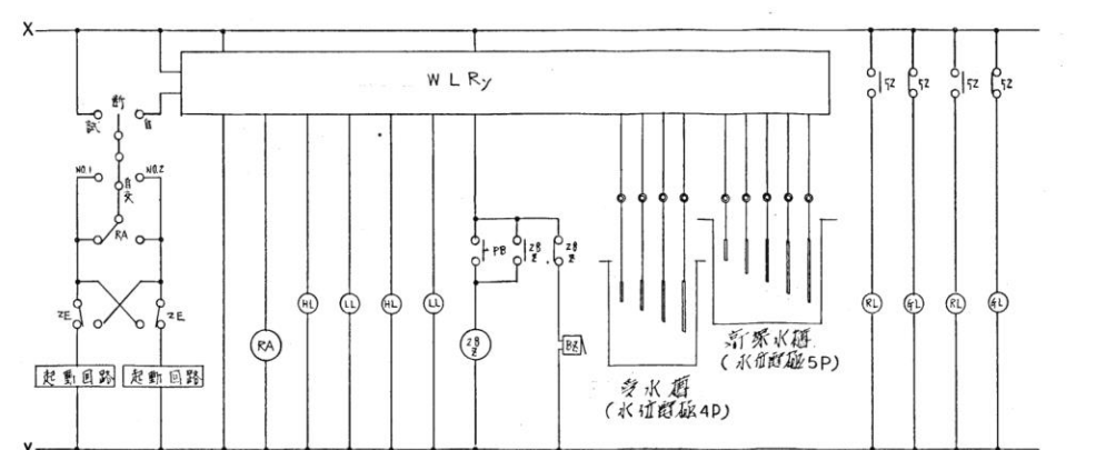
揚水ポンプ制御回路
