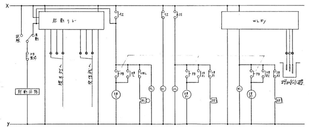
消火ポンプ制御回路
