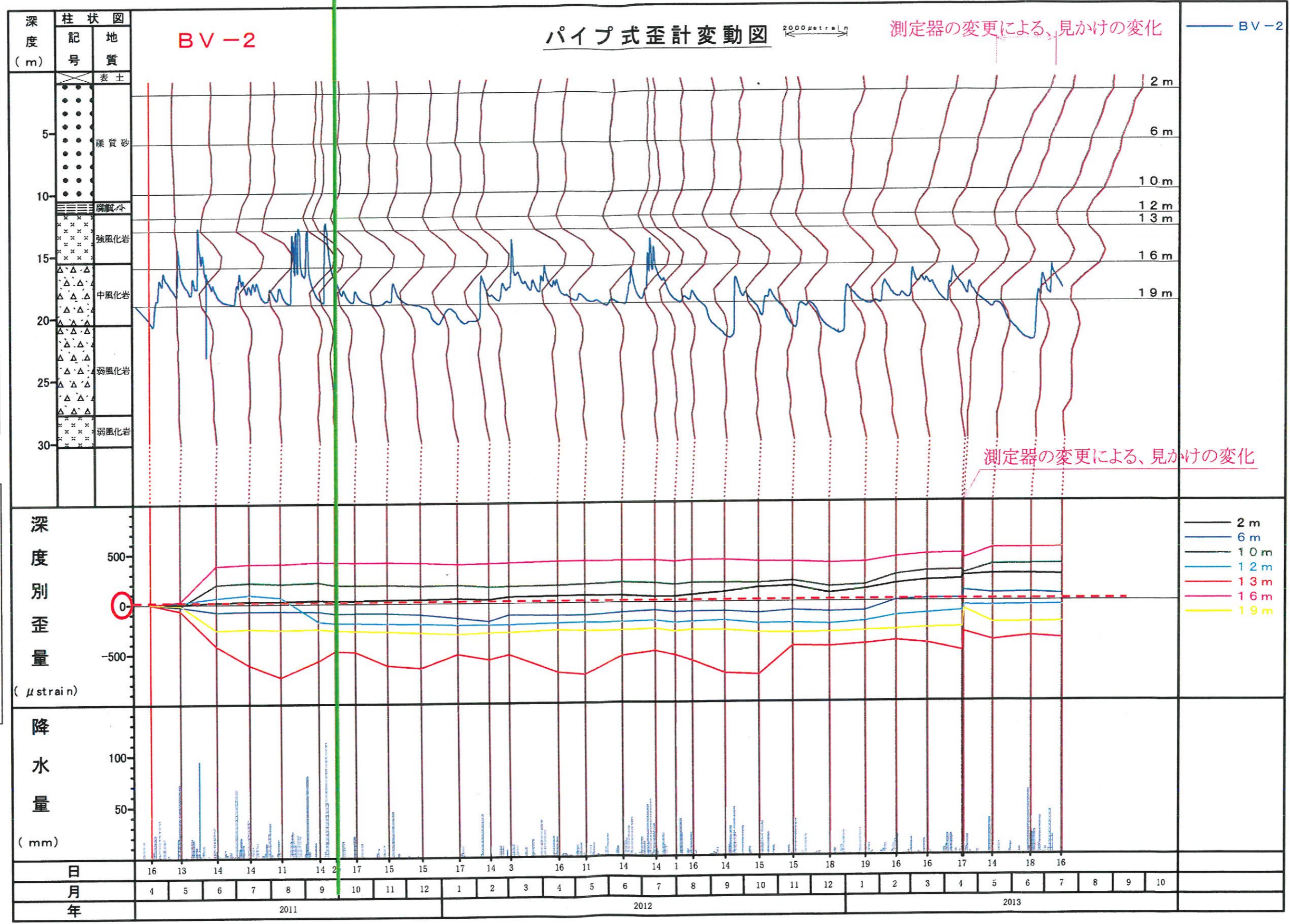
図-11 観測結果図 (BV-2)
