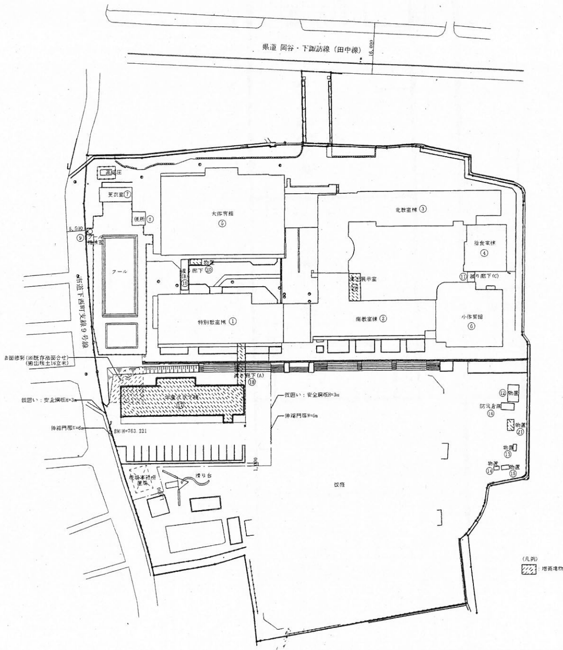
配置図 S=1/600
